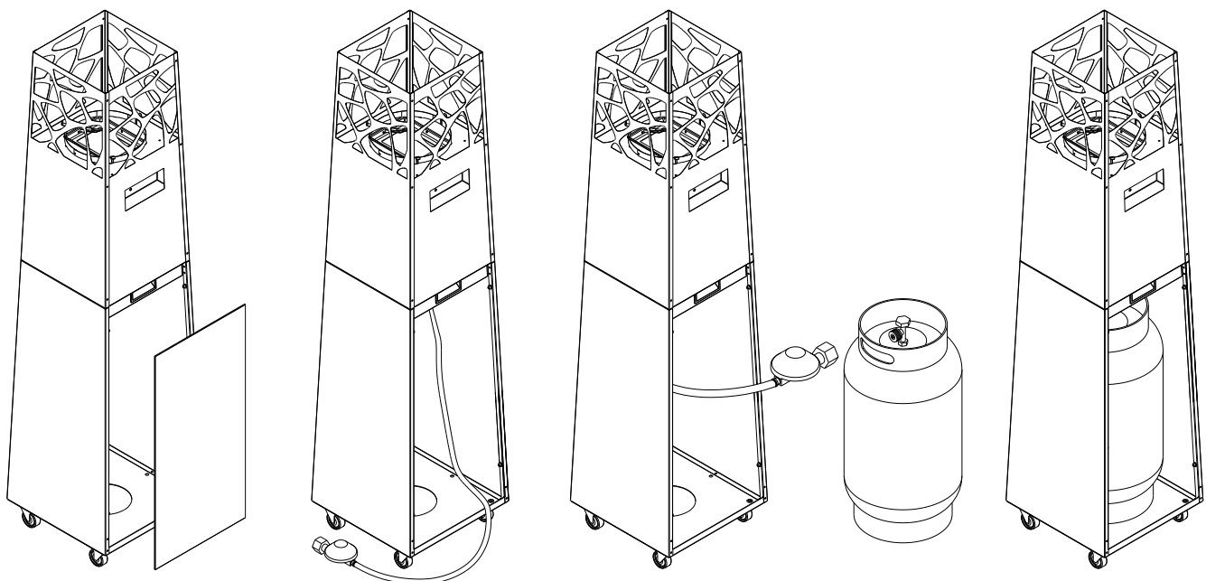
Abb. 9– Einbau der Gasflasche
