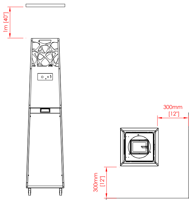
Fig 2 – Distancias mínimas
