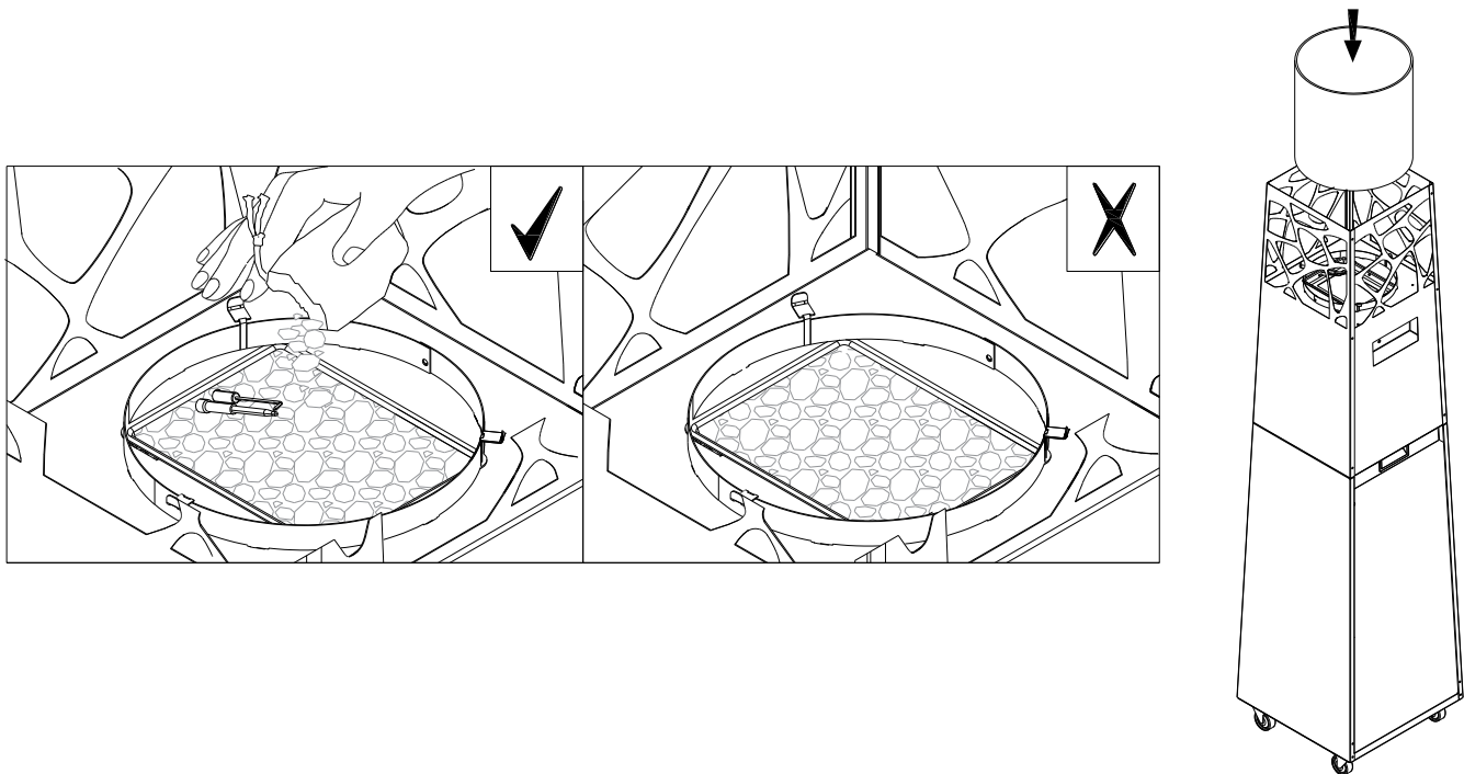
Abb. 8 – PYRAMID-Draufsicht mit Detailansicht der Zündelemente
