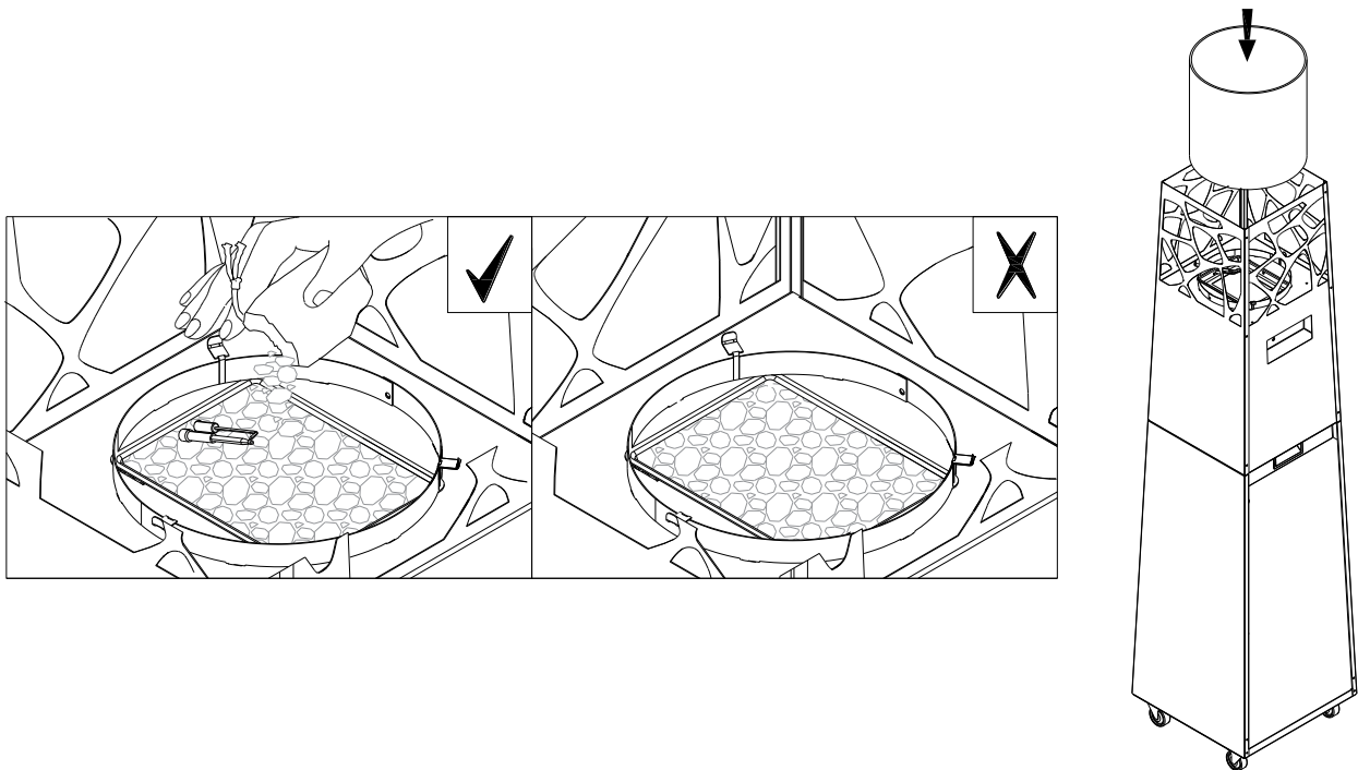
Fig. 8 – Vue de dessus de la PYRAMIDE avec détail des éléments d'allumage
