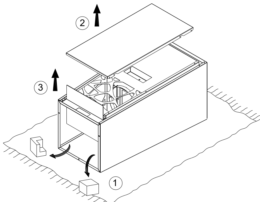
Rys. 4 – Rozpakowywanie kominka
