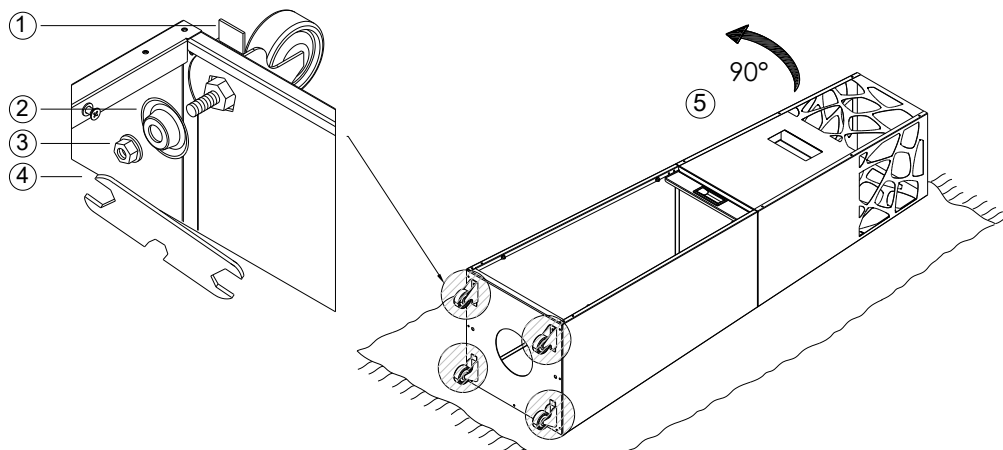
Fig. 7 – Installation des roues
