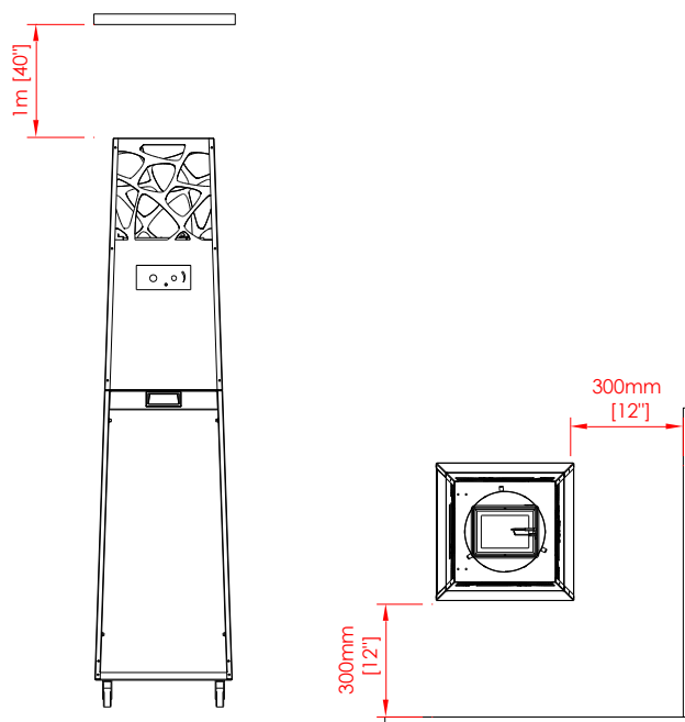
Fig 2 – Distanze minime
