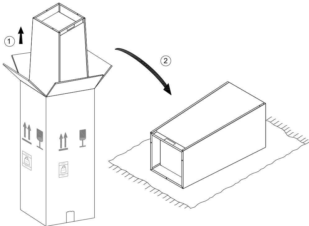
Abb. 3 – Auspacken des Kamins
