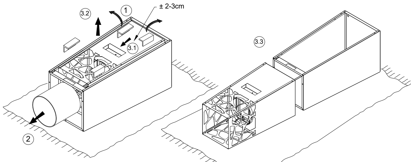
Abb. 5 – Auspacken des Kamins
