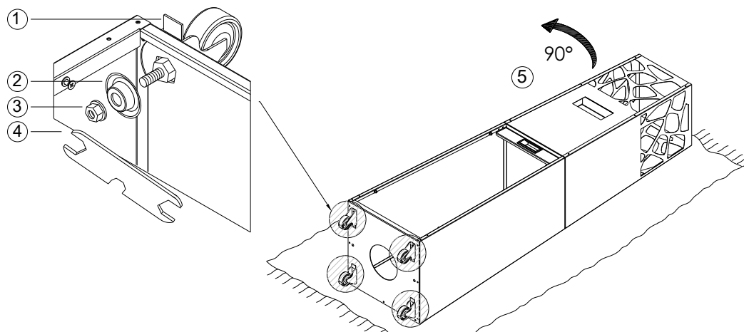
Fig. 7 – Instalación de las ruedas
