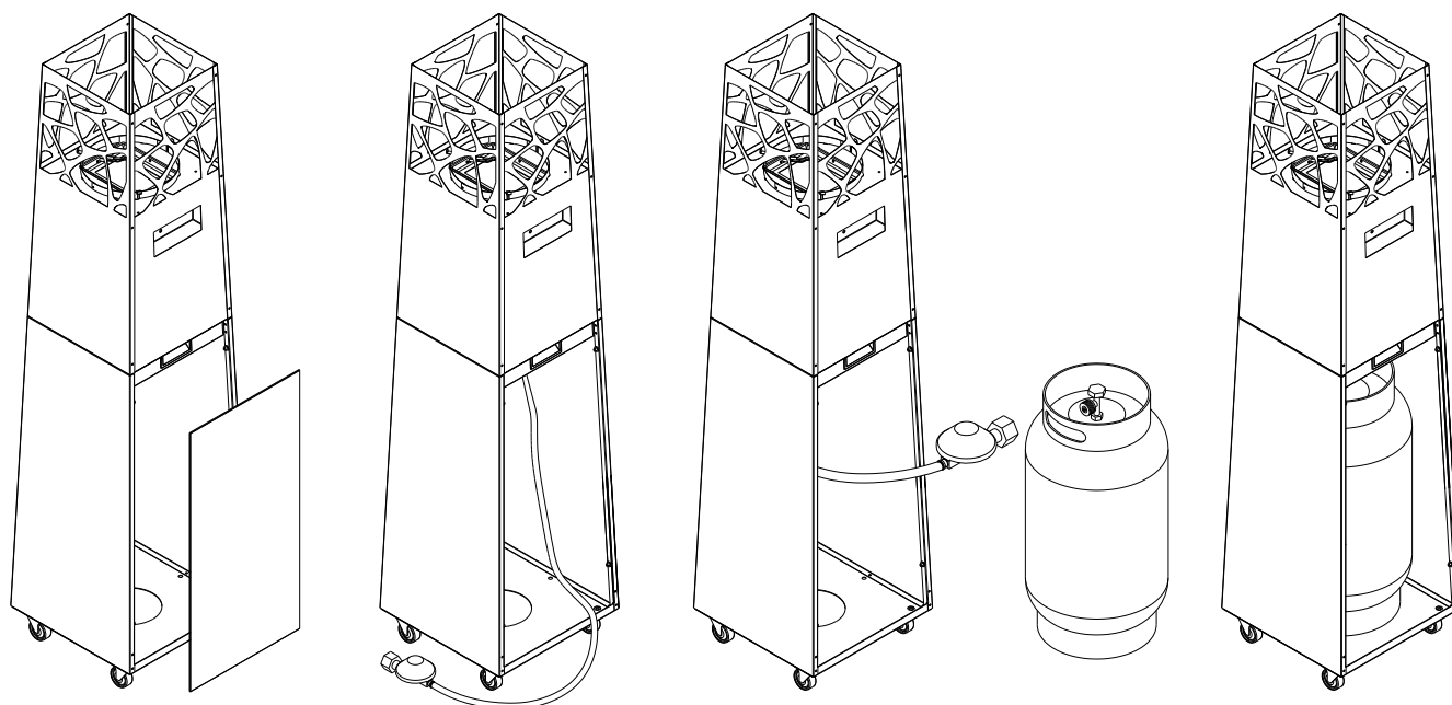
Rys. 9 – Montaż butli z gazem
