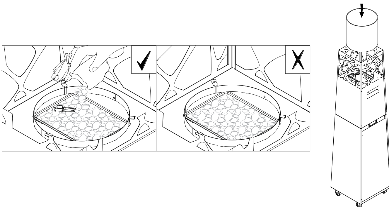
Fig. 8 - Vista dall'alto della PIRAMIDE con dettaglio degli elementi di accensione
