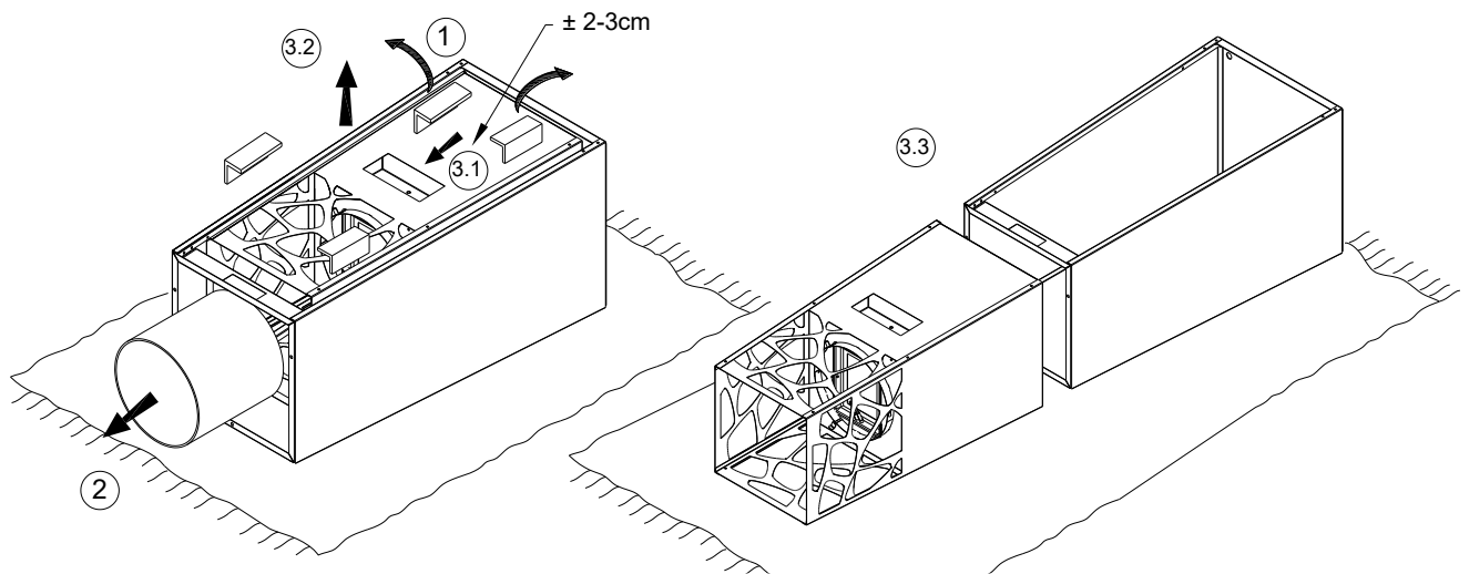
Fig. 5 – Déballage de la cheminée
