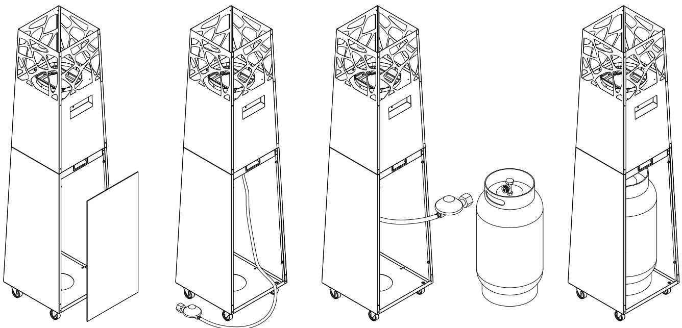
Fig 9– Installation de la bouteille de gaz
