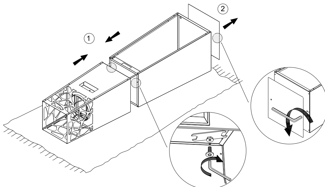
Rys. 6 – Łączenie części kominka i odkręcanie osłony ochronnej
