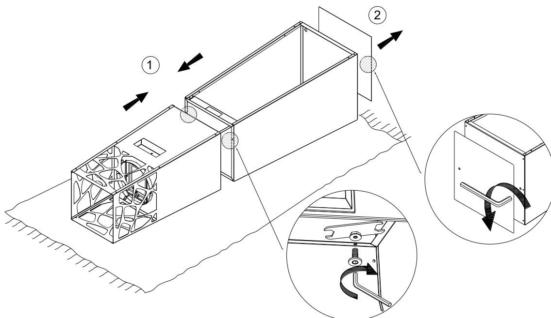
Fig. 6 – Unión de las piezas de la chimenea y desatornillado de la cubierta protectora
