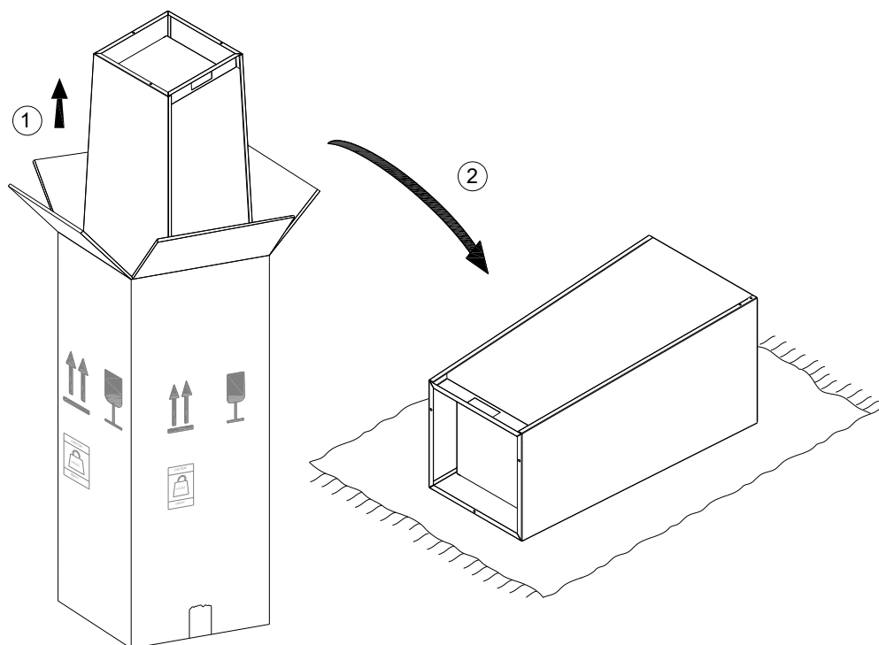
Fig. 3 – Déballage de la cheminée
