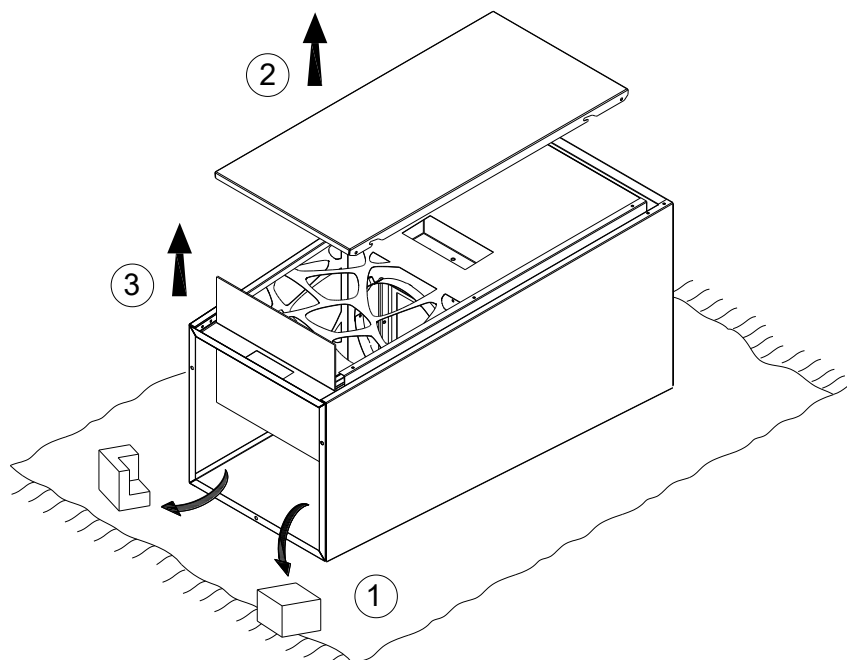
Fig. 4 – Déballage de la cheminée
