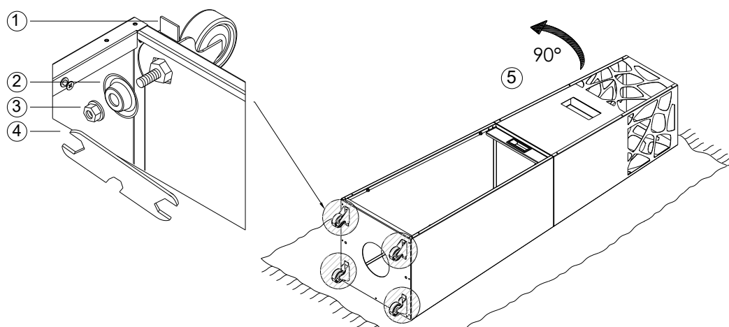
Abb. 7 – Einbau der Räder
