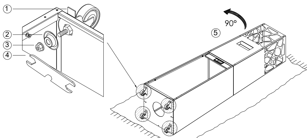
Fig. 7 - Montaggio delle ruote
