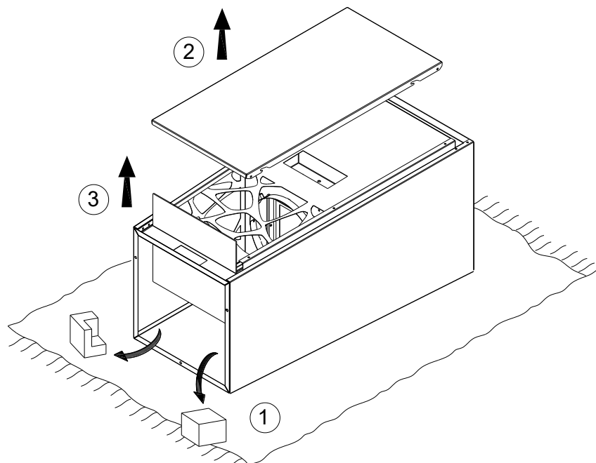
Abb. 4 – Auspacken des Kamins
