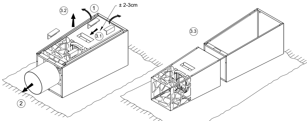
Rys. 5 – Rozpakowywanie kominka
