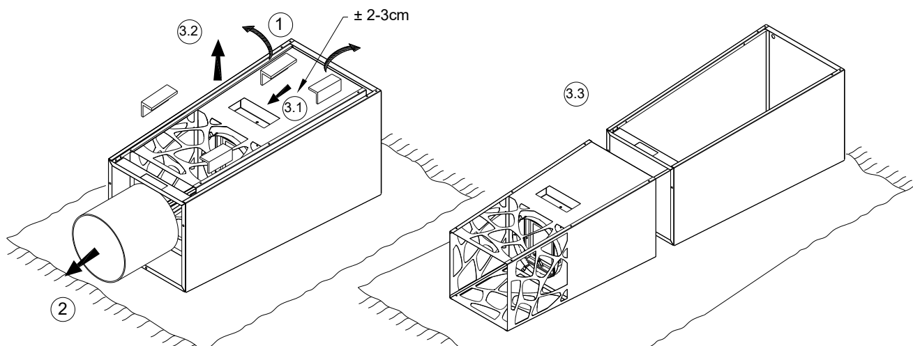
Fig. 5 – Desembalaje de la chimenea
