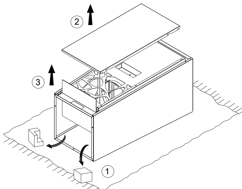
Fig. 4 – Desembalaje de la chimenea
