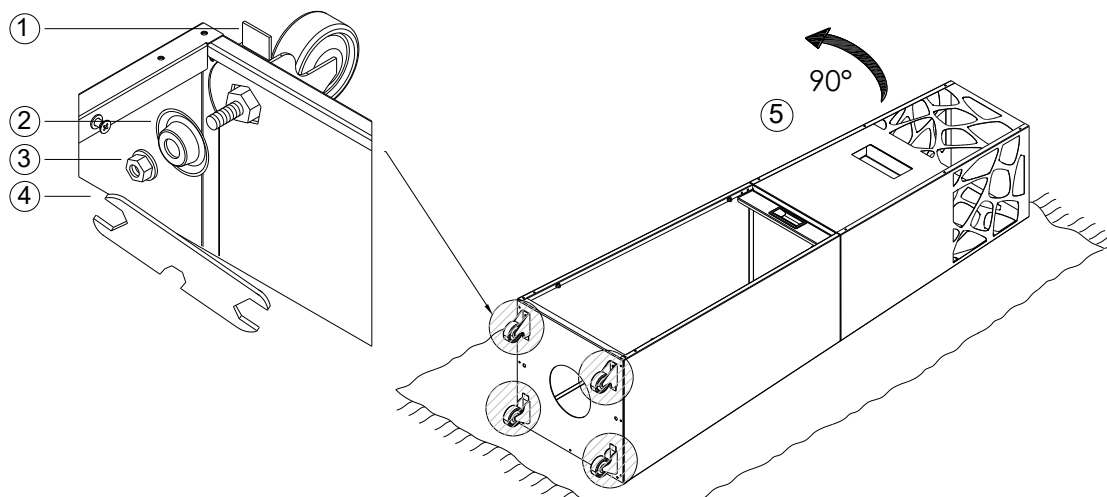
Rys. 7 – Montaż kół
