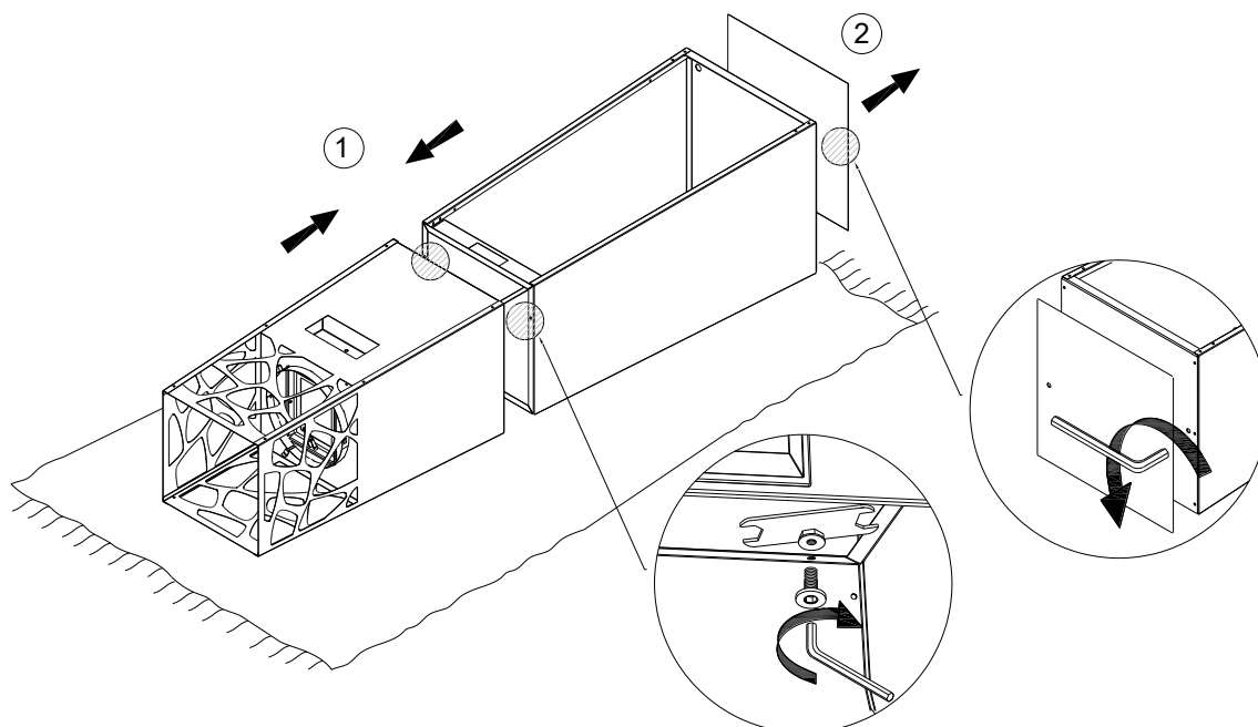
Abb. 6 – Verbinden der Kaminteile und Abschrauben der Schutzabdeckung
