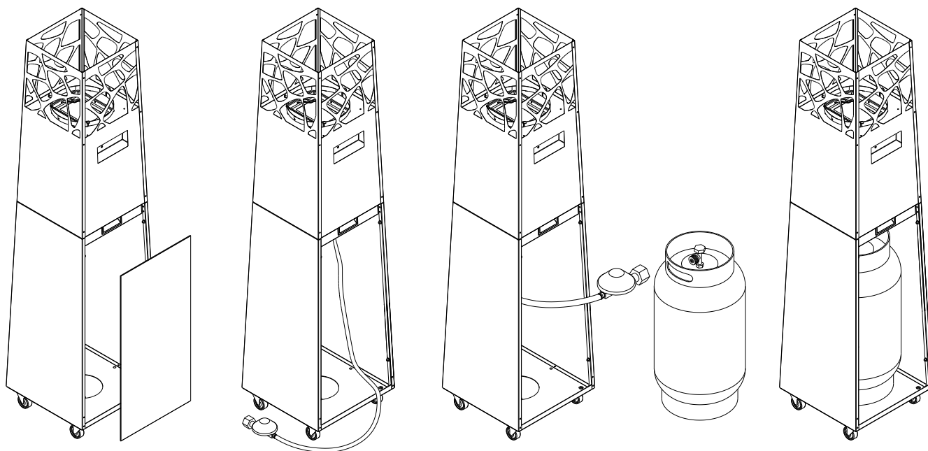
Fig 9– Instalación de la bombona de gas
