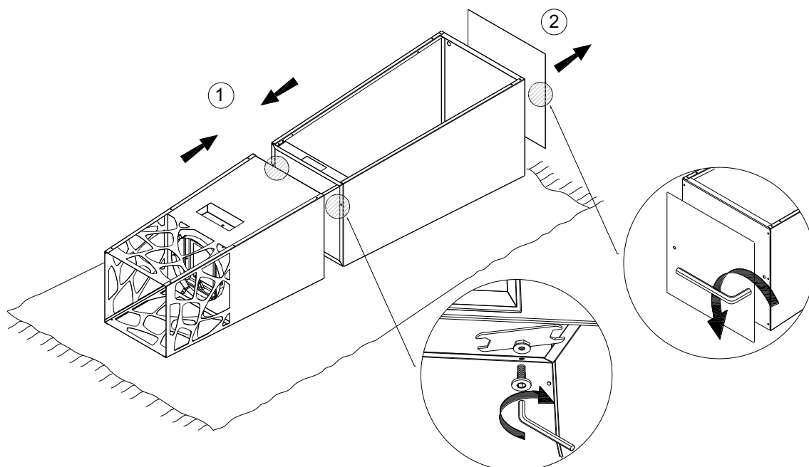
Fig. 6 - Collegamento delle parti del caminetto e svitamento del coperchio di protezione
