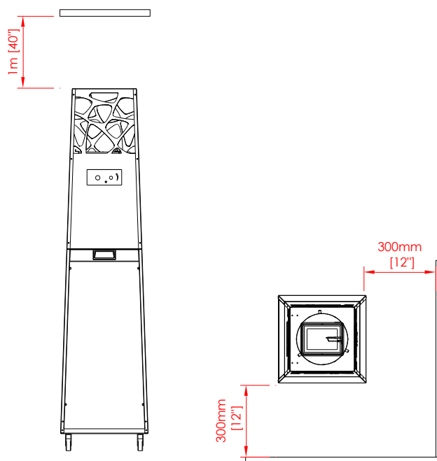
Rys. 2 – Odległości minimalne
