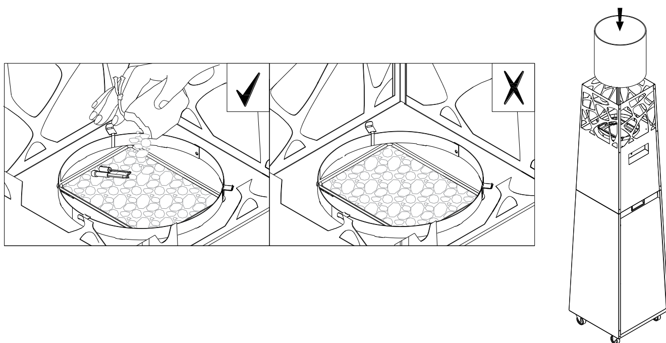
Fig. 8 – Vista superior de PYRAMID con detalle de los elementos de encendido
