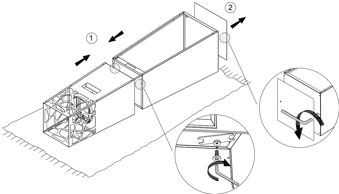
Fig. 6 – Assemblage des pièces du foyer et dévissage du couvercle de protection
